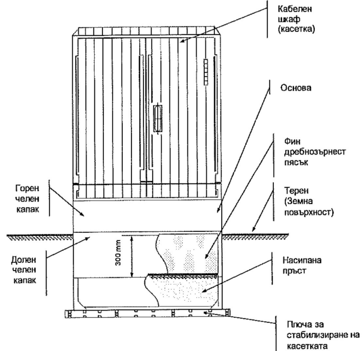
Фигура – Монтаж на пластмасов разпределителен шкаф (касета)
